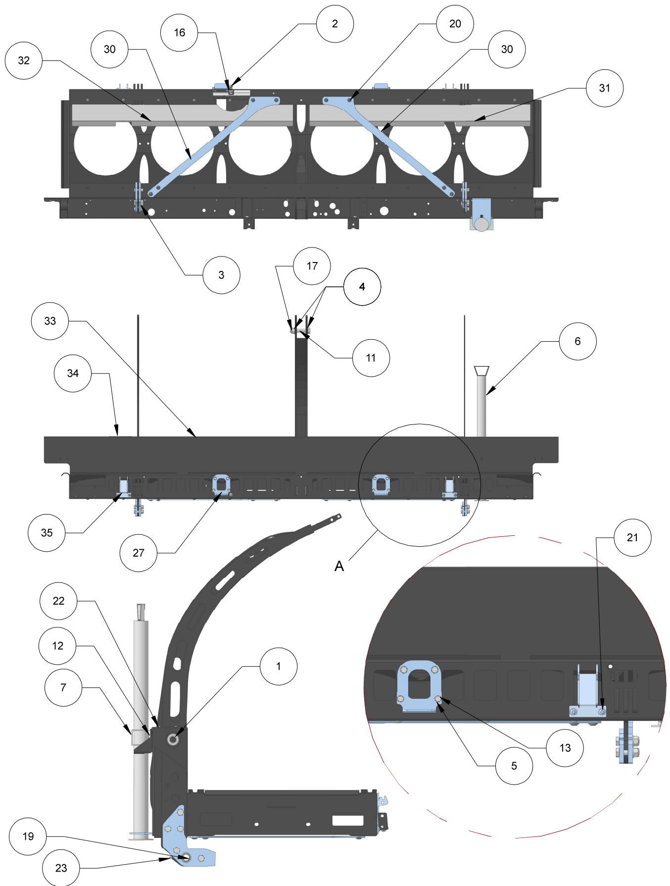
Detailansicht A
